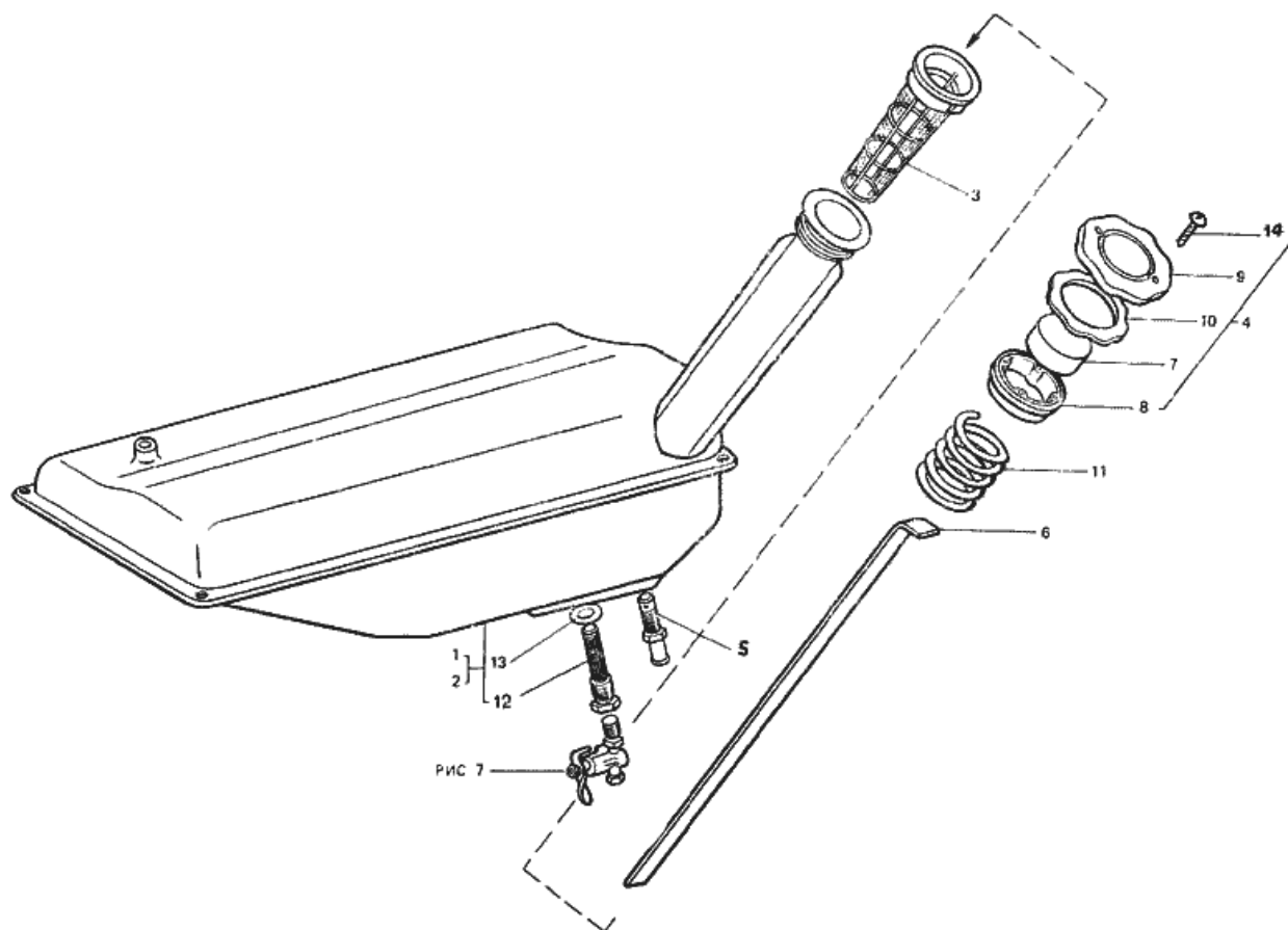
Рис. 66. Бак топливный Т40-1100650-Б, Т40АН-1100050
